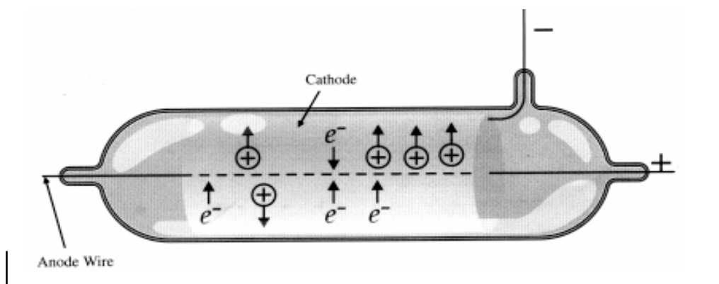
Geiger-Muller Tube
